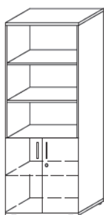
MR-2 80x40x187
